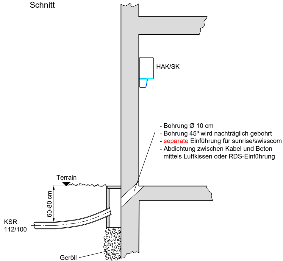
Schnitt
