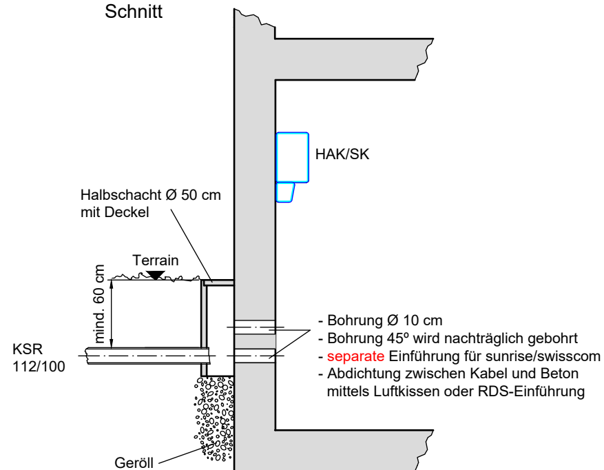
Schnitt
