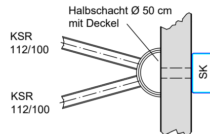
Draufsicht
