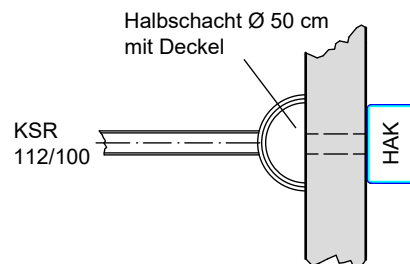
Draufsicht
